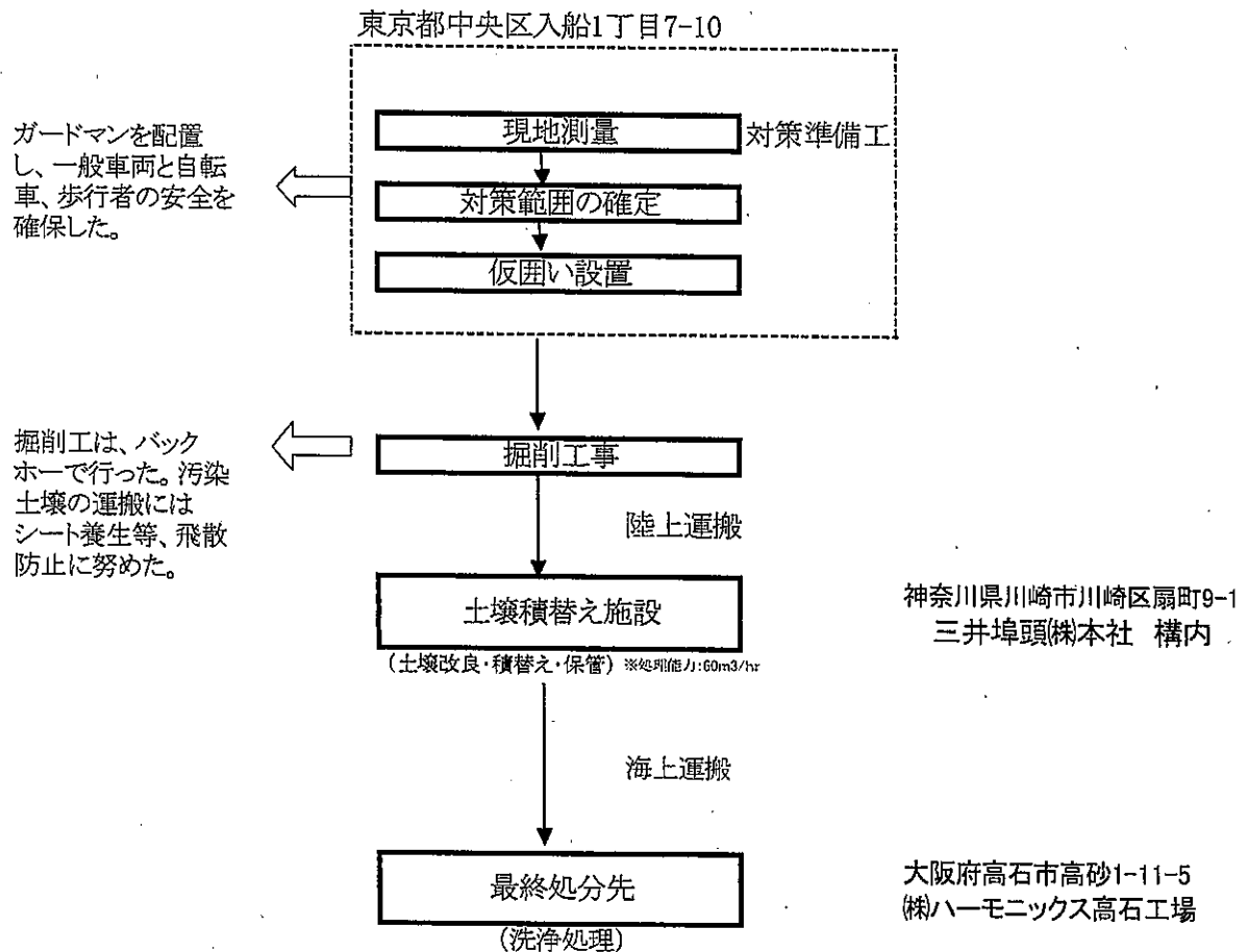
【汚染土壌処理フロー図】
