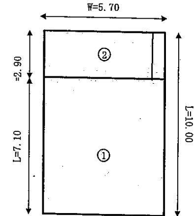
平面図
