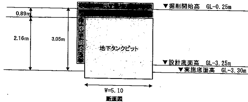
断面図
