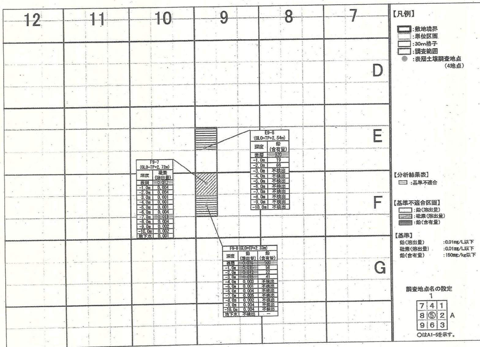
図 7-2 土壌汚染状況平面図
