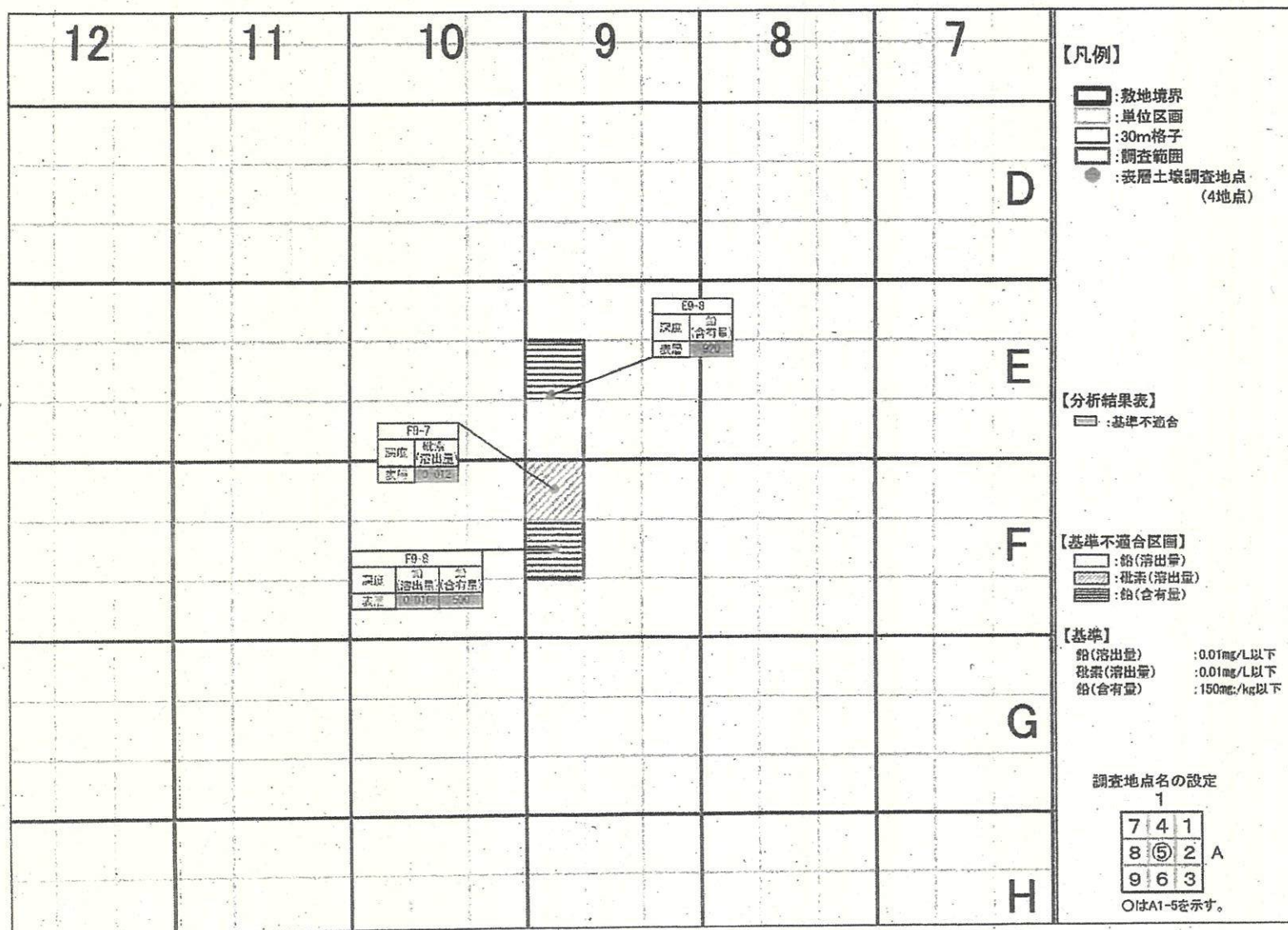
図 5-1 土壌汚染状況図
