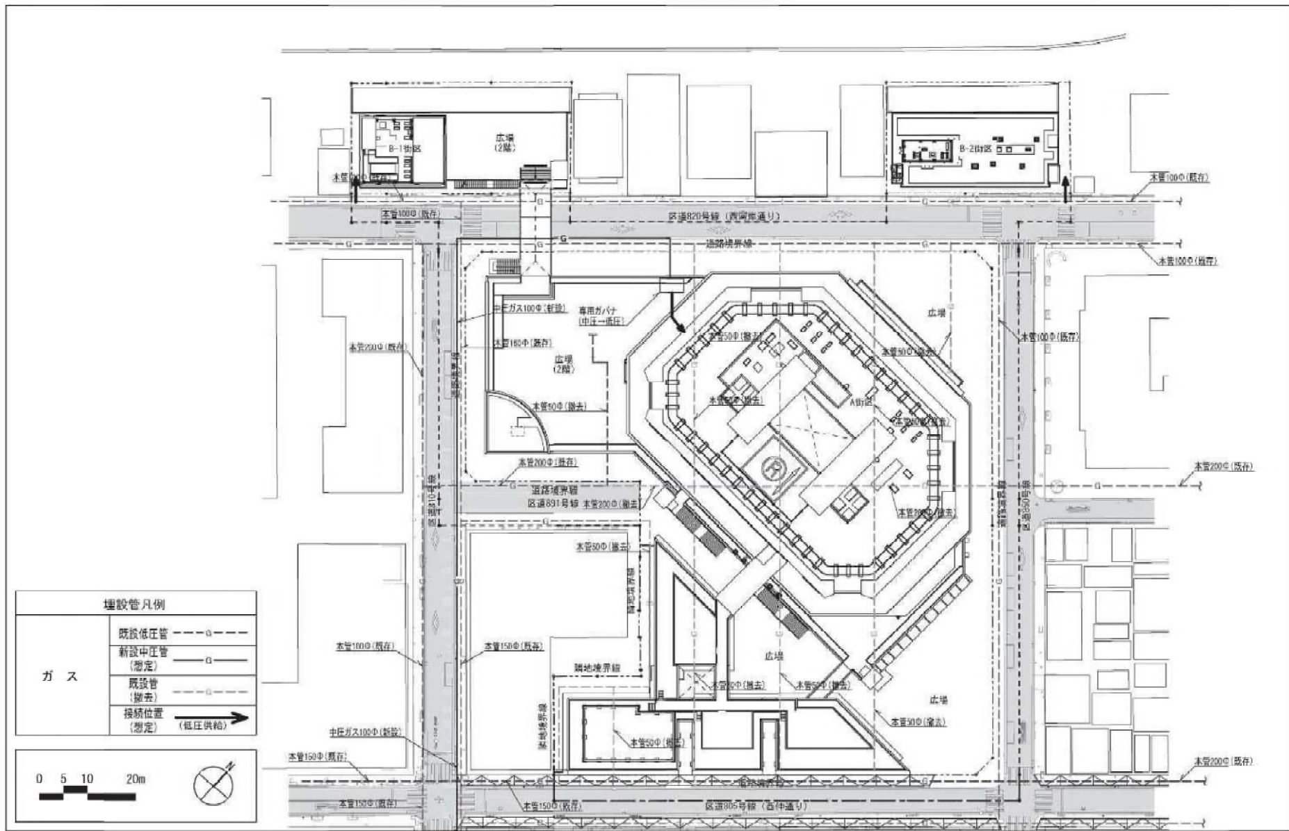
月島三丁目北地区第一種市街地再開発事業 3-2) 施設建築敷地の設計図 ガス計画平面図 S=1/500 (A2)
