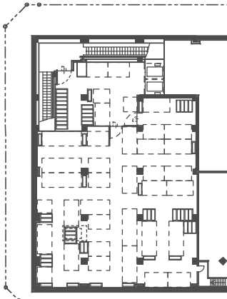
地下1階
