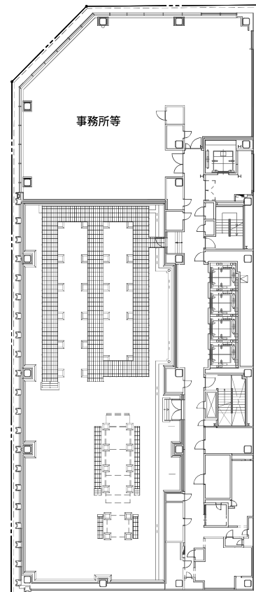
10階平面図 1/500
