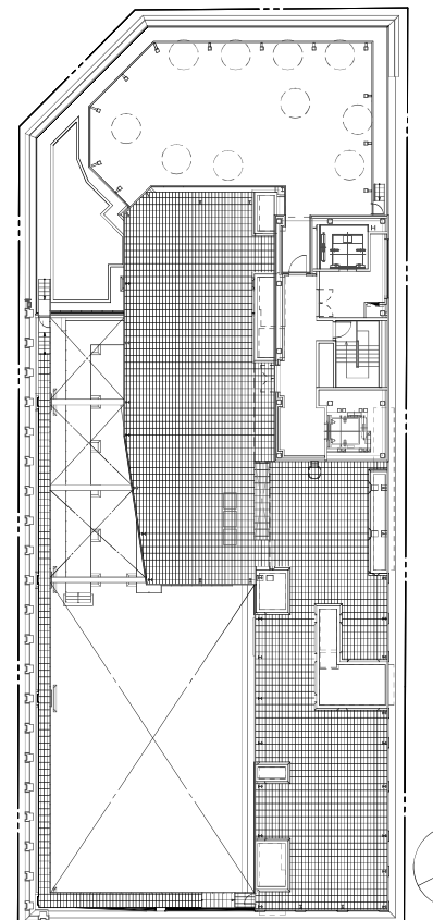
RF平面図 1/500
